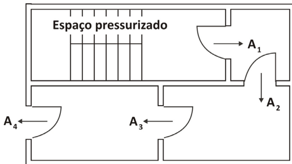
Figura 2 - Trajetórias de escape do ar em série
